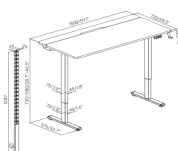
Dimenziók (mm/col)
